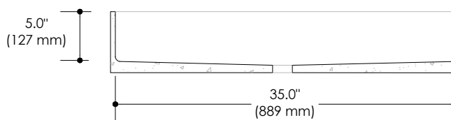
COUPE A
