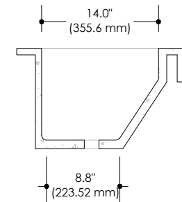
COUPE B
