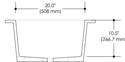
COUPE A
