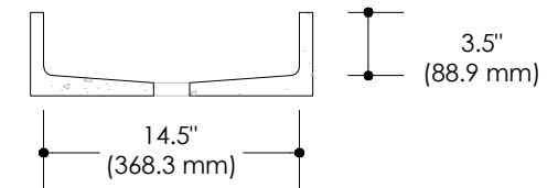
COUPE B
