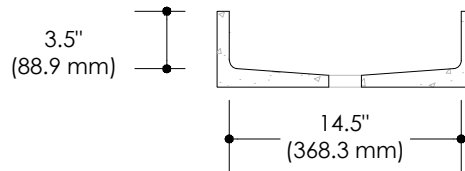
COUPE A
